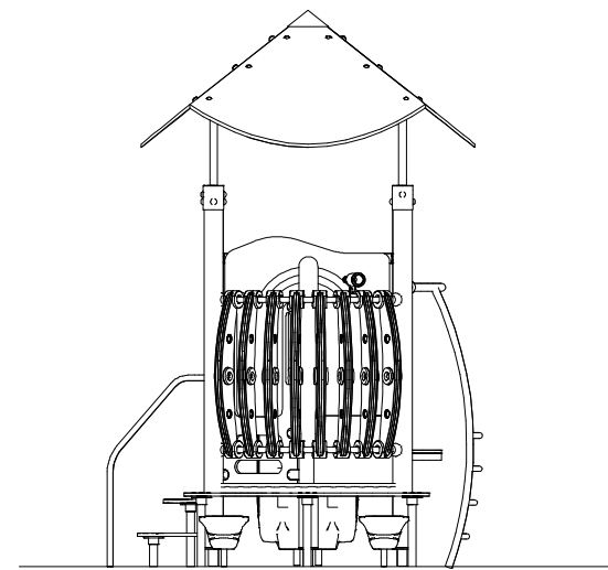
ELEVATION - RIGHT
