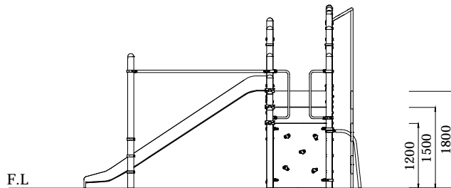
ELEVATION - RIGHT
