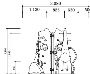
ELEVATION - RIGHT
