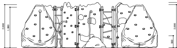
ELEVATION - RIGHT
