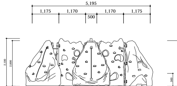
ELEVATION - RIGHT
