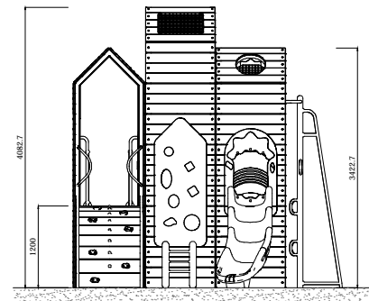
ELEVATION - RIGHT
