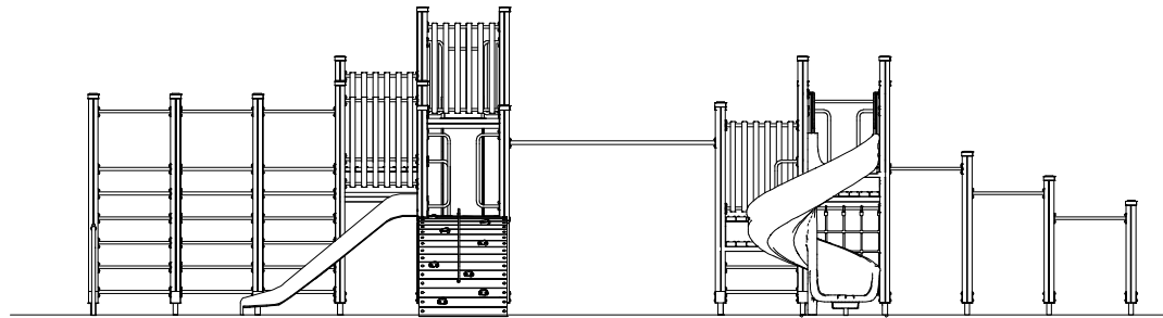
ELEVATION - RIGHT
