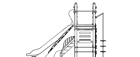
ELEVATION - RIGHT
