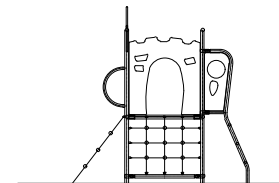
ELEVATION - RIGHT
