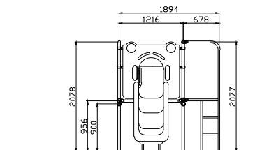
ELEVATION - RIGHT
